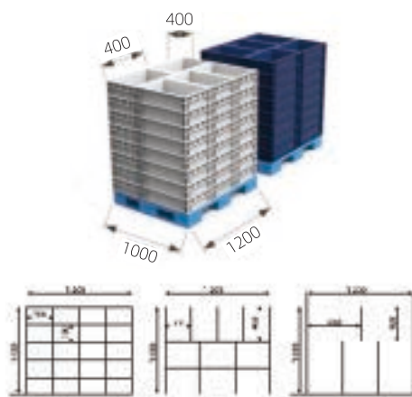
国际通用标准EU周转箱完美配合标准托盘
